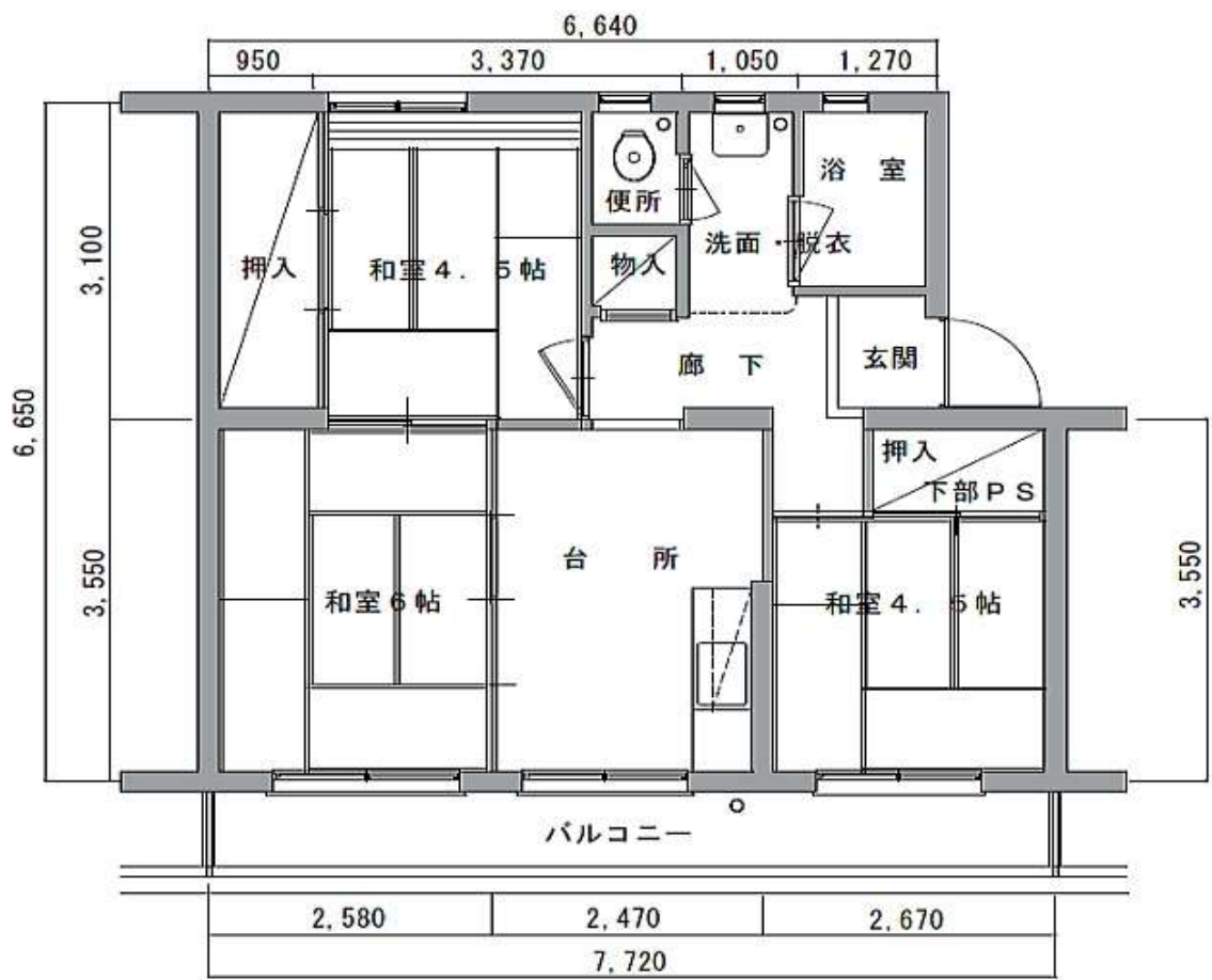
公社賃貸住宅 共通間取り平面図(南橋・大和根・広瀬・井野)
