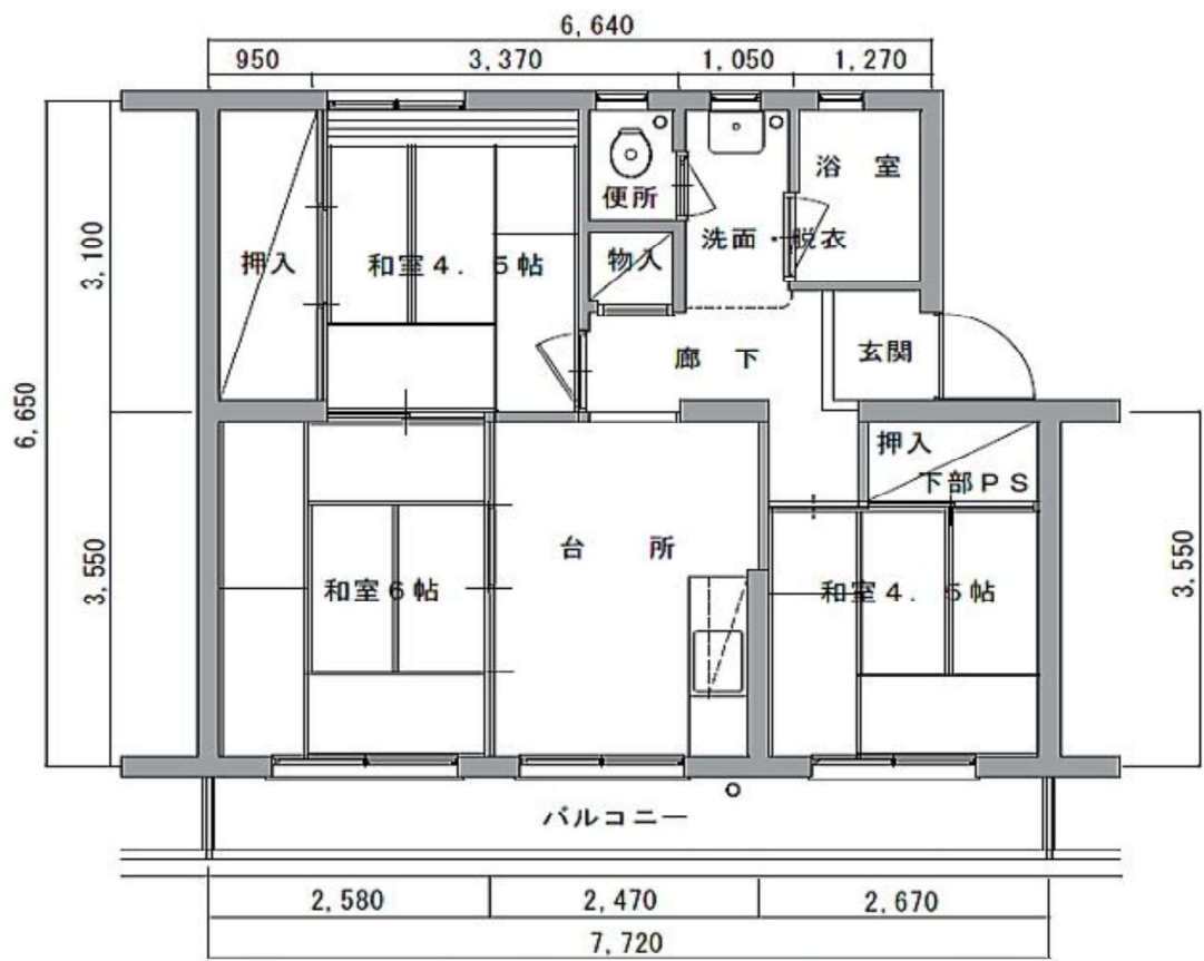
公社賃貸住宅 共通間取平面図(南橋・大利根・広瀬・井野)
