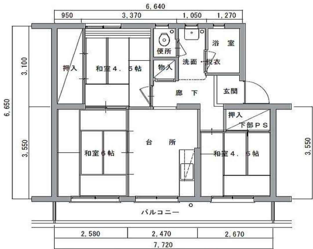
公社賃貸住宅 共通間取り平面図(南橋・大和根・広瀬・井野)
