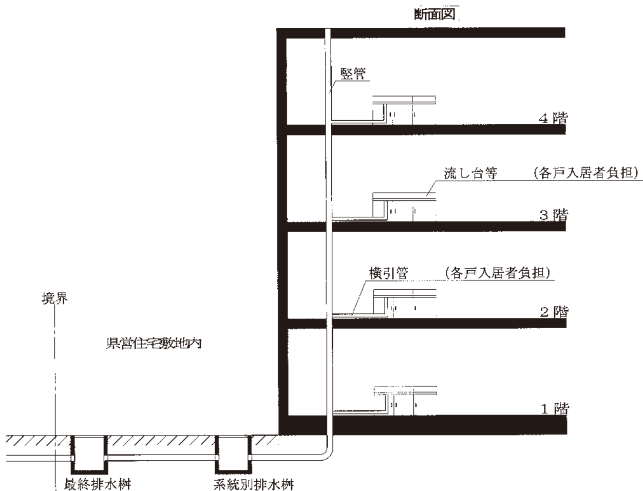
図-7 排水管系統図 (原因が入居者にある場合) ※各排水系統でつまった場合はその排水管系統 を使用している4戸で等分の負担となります。 ※建物最終樹までの配管でつまった場合は その建物全戸で等分の負担となります。
